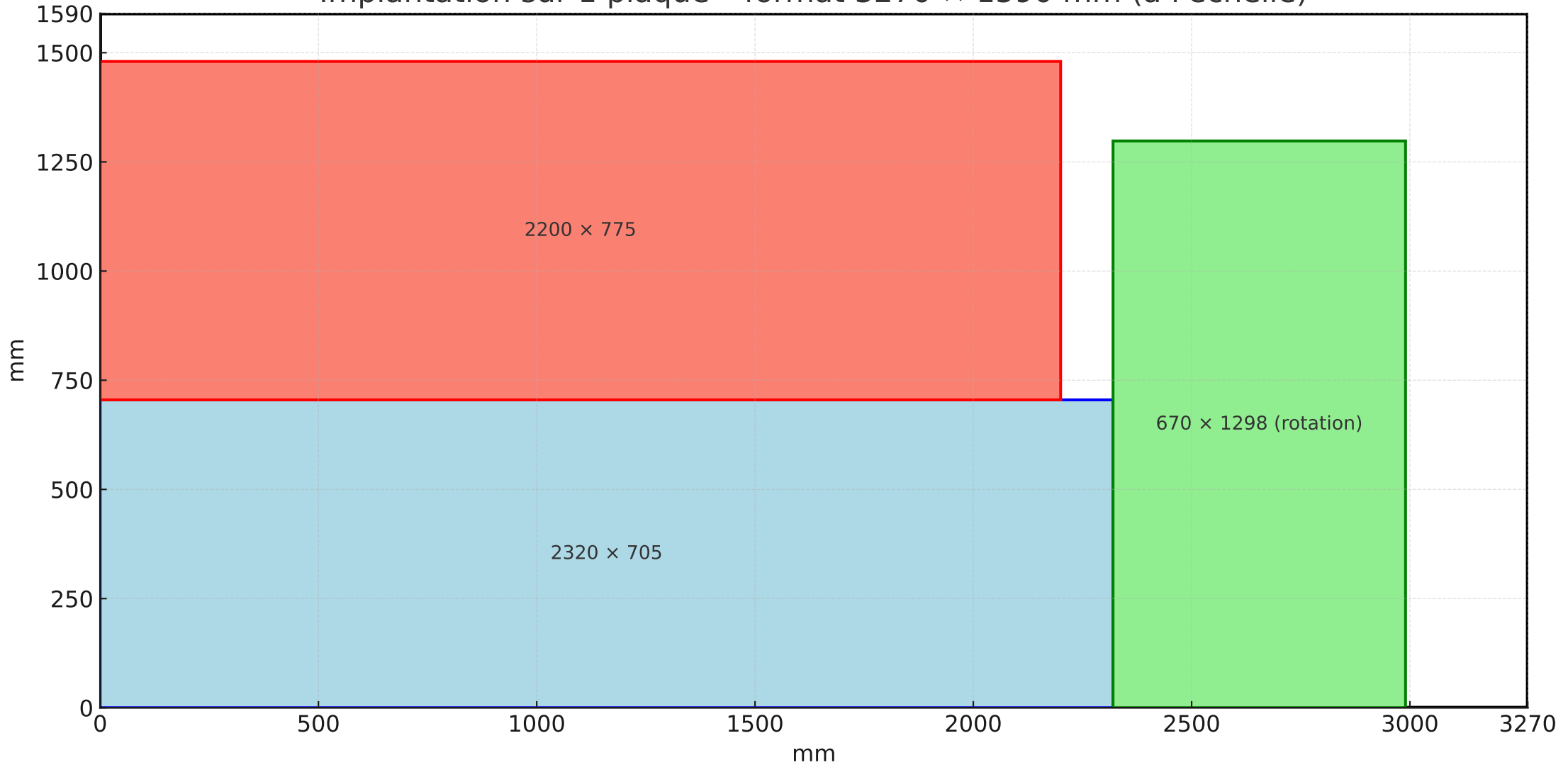
Implantation sur 1 plaque - format 3270 × 1590 mm (à l'échelle)
